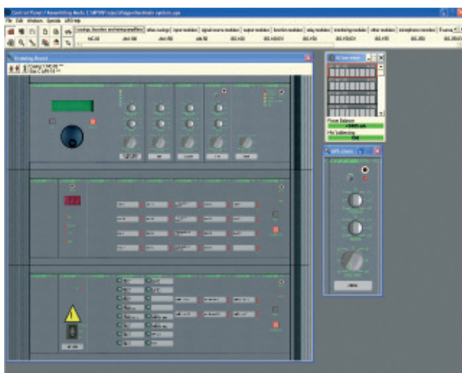
Virtueller Hardware-Aufbau des kompl. Systems durch Drag and Drop.
