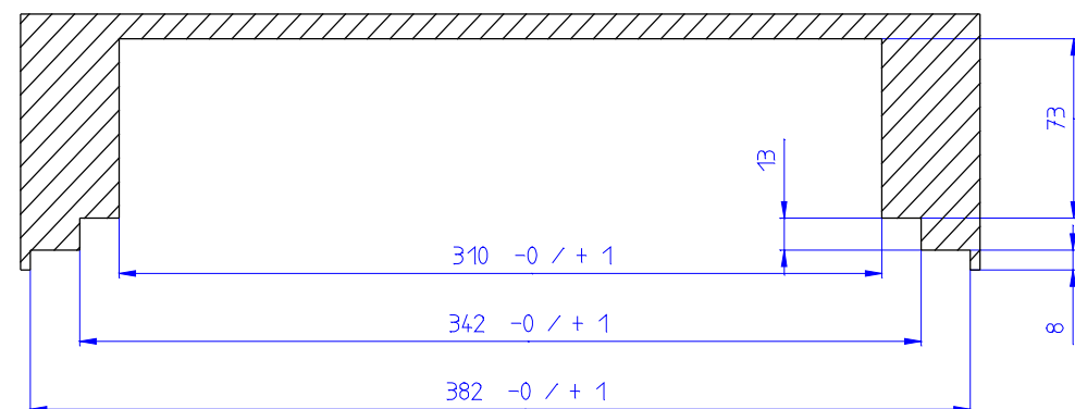
schnitt B-B
